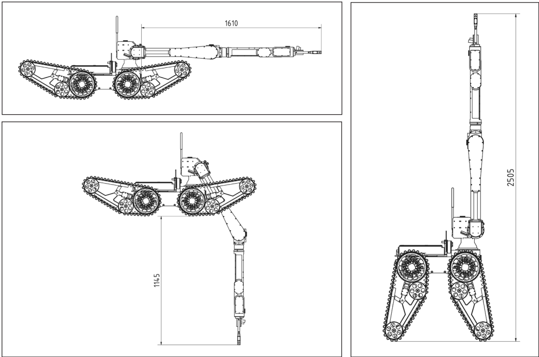
Abbildungen: Reichweite
