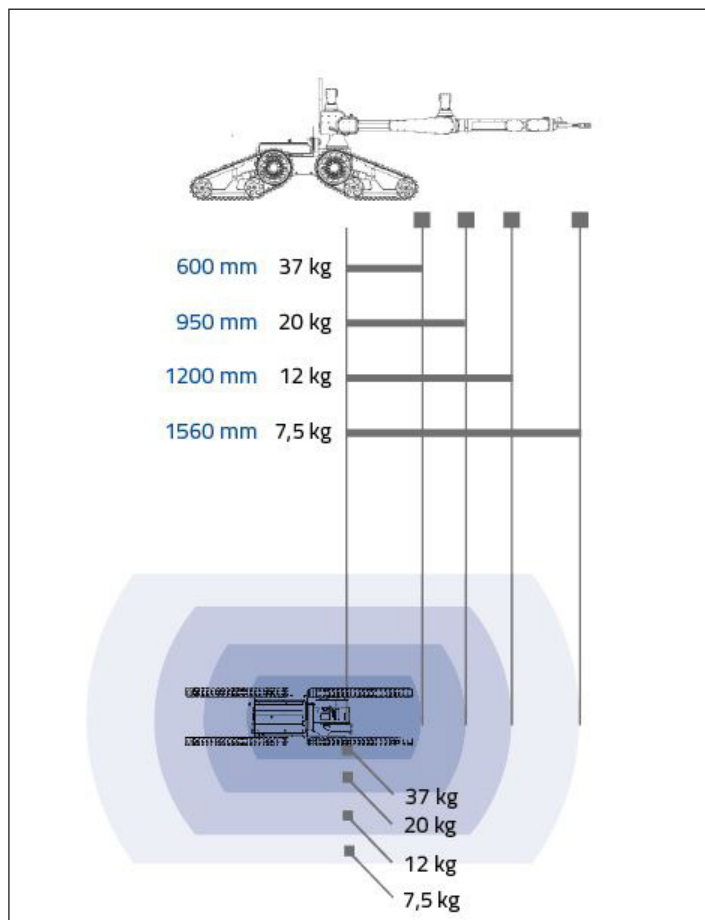
Abbildung: Lastdiagramm
