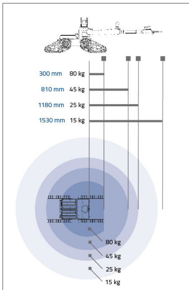
Abbildung: Lastdiagramm
